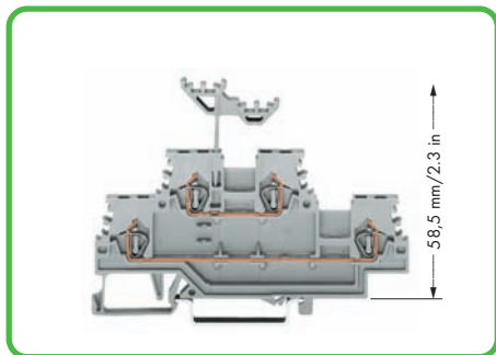
Двухуровневый маркировочный адаптер Высота включает двухуровневый маркировочный адаптер WSB
